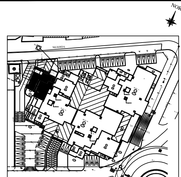
PLAN MASSE
