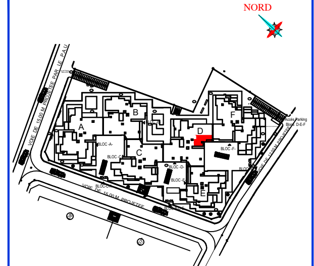
PLAN MASSE
