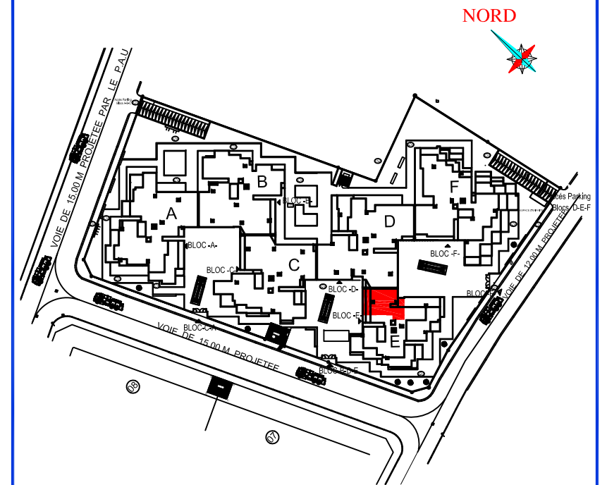
PLAN MASSE
