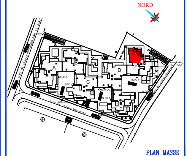
PLAN MASSE
